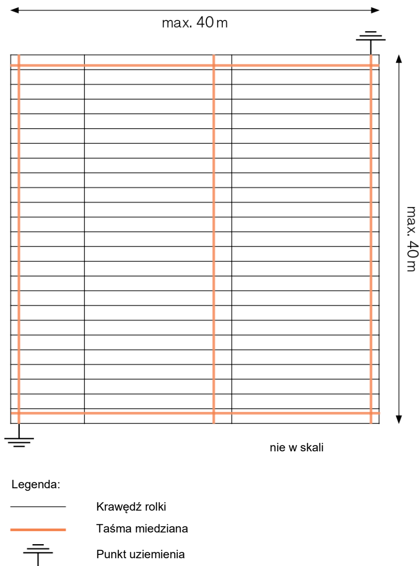
Rys. 2 - Przykład przewodzącej i rozpraszającej energię instalacji rolek noraplan ® ec/ec na dużych obszarach:
