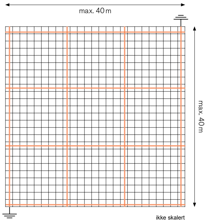
Fig. 3 – Eksempel på ledende og avledende legging av noraplan ® ed/ec fliser for store områder:
