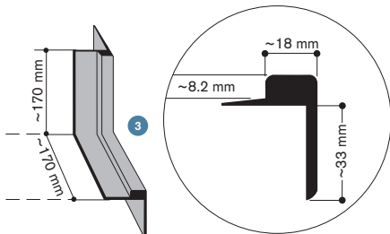
Plinthes à crémaillère nora® TG 7003 U (Angle rentrant)
