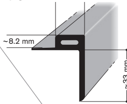
Bordure de finition nora® A 5013 U
