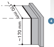
Plinthes à crémaillère nora® TG 7004 U (Angle sortant)
