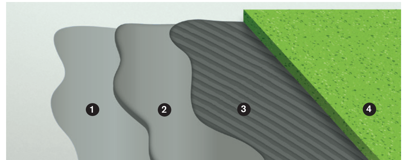
Le système nora one — 1 Primaire 2 Ragréage 3 Colle 4 Revêtement de sol en caoutchouc nora
