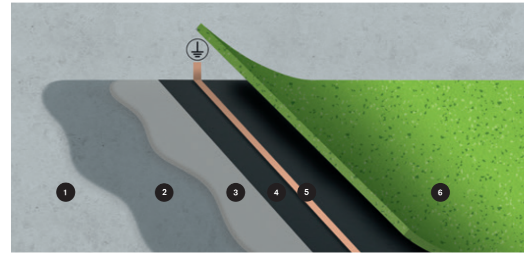
1 基层 2 界面剂 3 自流平 4 诺拉 dryfix ed 5 铜条 6 诺拉® ESD 静电防护地板
