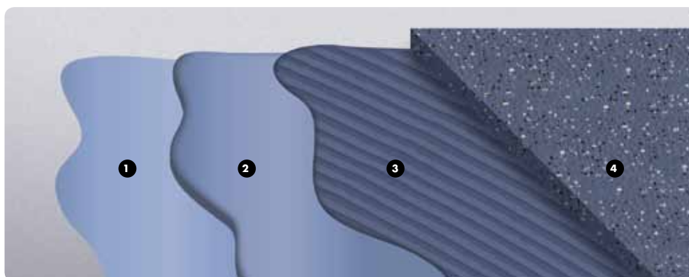
Structure du système : 1 Primaire 2 Ragréage 3 Colle 4 Revêtement de sol
