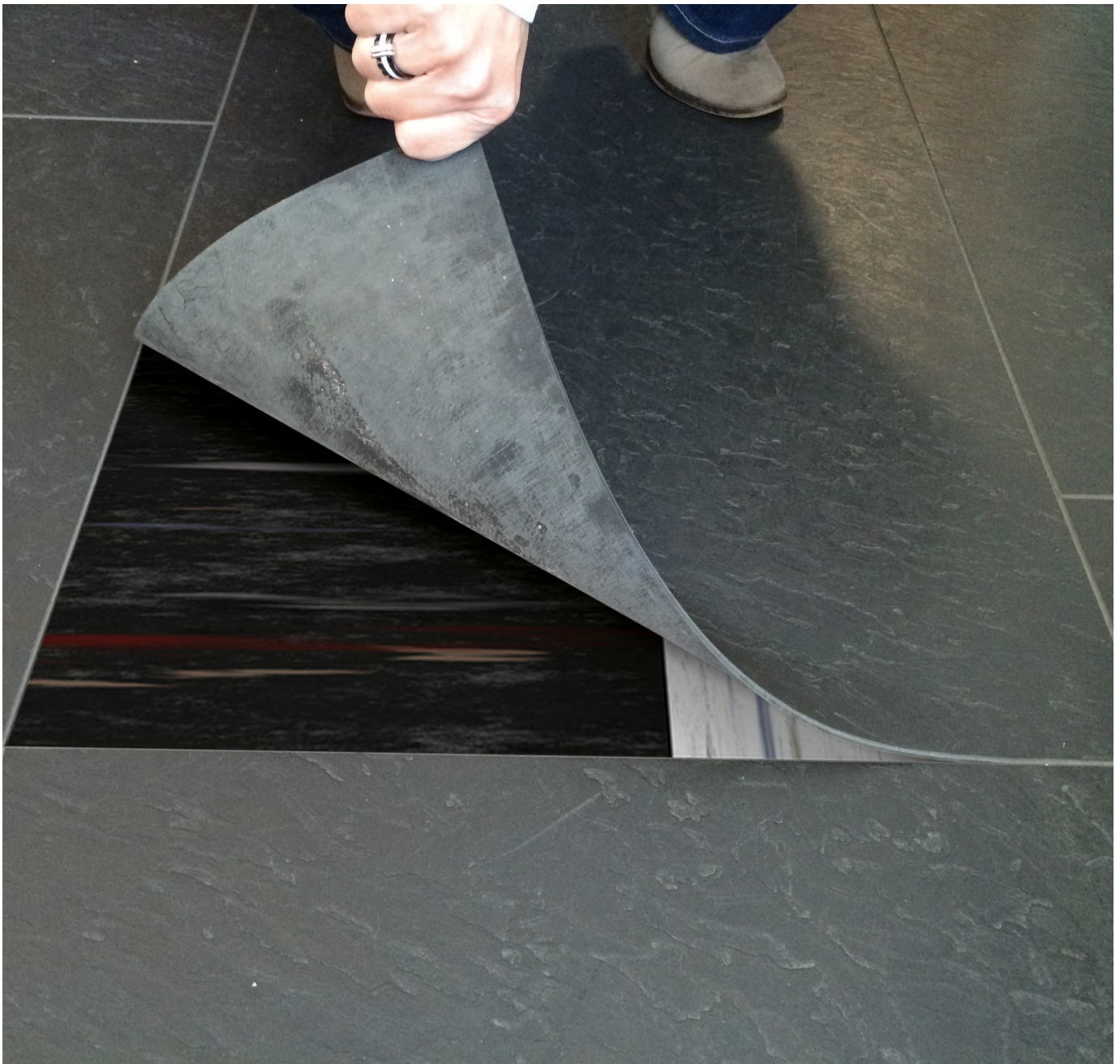
Pose rapide sur d'anciennes dalles vinyles amiantées
