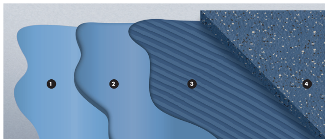
Structure du système : 1 Primaire 2 Ragréage 3 Colle 4 Revêtement de sol. Chaque élément répond à des critères écologiques.
